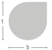
STAHLBODENPLATTE Tropfen | grau
